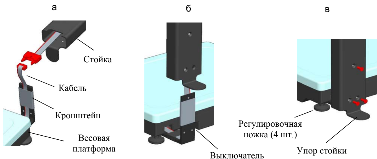
Рис. 4. Сборка
