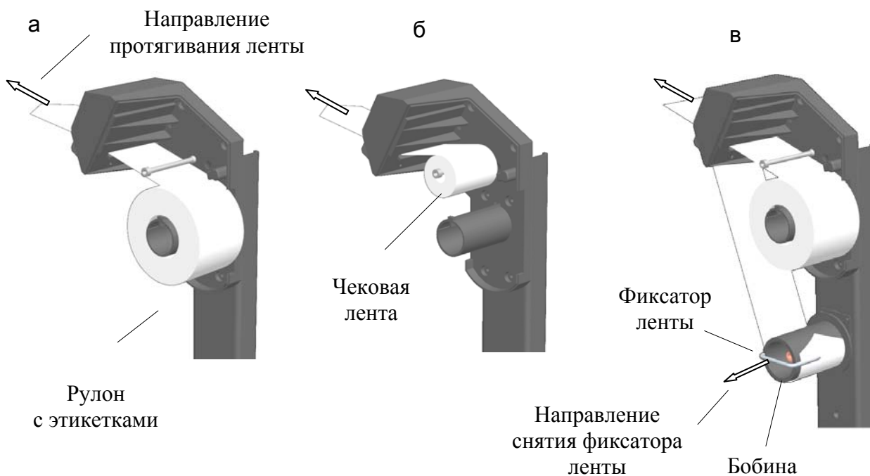
Рис. 6. Установка рулонов
